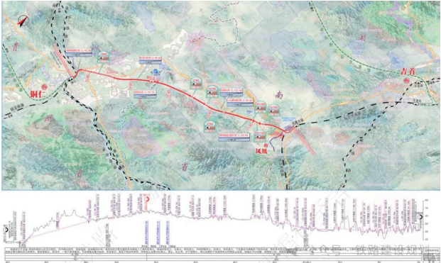
铜吉铁路线路平纵断面示意图。
